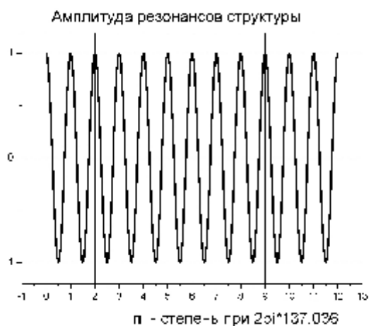
Рис.15 Резонансы структуры вакуума согласно таблице 3.
